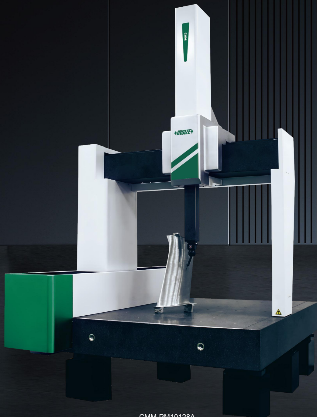
CMM-PM10128A
